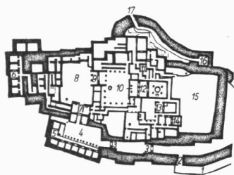
Тиринф. План крепости: 1 — наклонный въезд; 2 — внешние ворота; 3 — внутренние ворота (между ними тюрьма); 4 — передний двор; 5, 6 — казармы; 7 — внешние пропилеи; 8 — внешний дворцовый двор; 9 — внутреннее пропилеи; 10 — внутренний дворцовый двор; 11 — баня; 12 — мегарон с тронном; 13, 14 — небольшие мегароны; 15 — средняя крепость; 16 — башня; 17 — западные ворота
